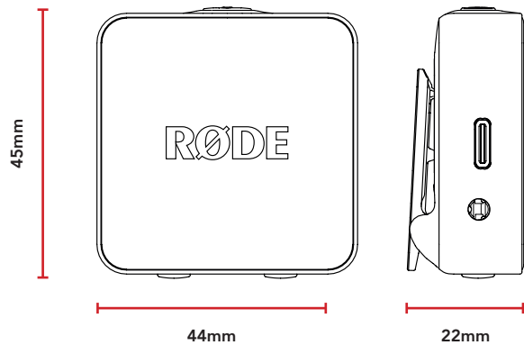
接收器(RX)
